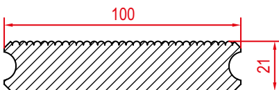
Thermo-Esche 21 x 100 mm, eins. fein geriffelt, eins. glatt gehobelt, seitlich mit Seno-Profil
