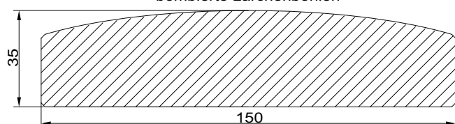
bombierte Lärchenbohlen
