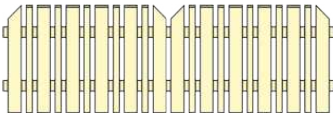
Beispiel 3: Vierkant-Zaunlatten 2,5 x 9,5 cm, Prog-Nr. 4095 kombiniert mit Zaunlatten 2,5 x 4,5 cm und 2,5 x 9,5 cm oben schräg abgebildetes Zaunfeld: 250 x 80 cm (L x H), Lattenabstand ca. 4 cm
