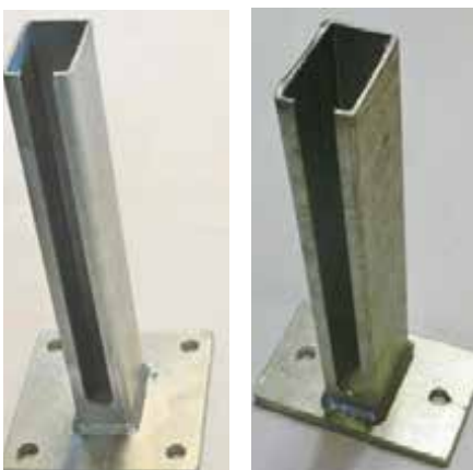
Pfostenhalter zum Aufdübeln (4)
