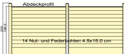
Lärmschutzwand "Spitzstein"
